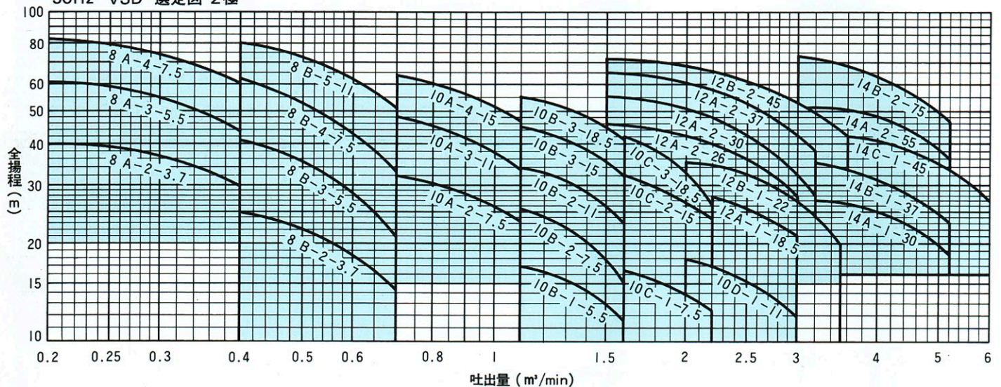
50Hz VSD 仕様・寸法表
