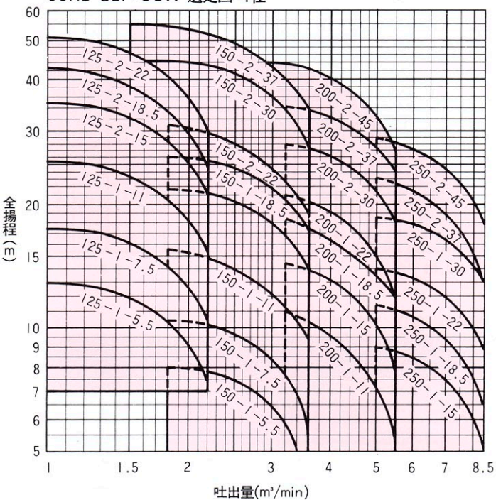
60Hz SSP・USW 仕様表
