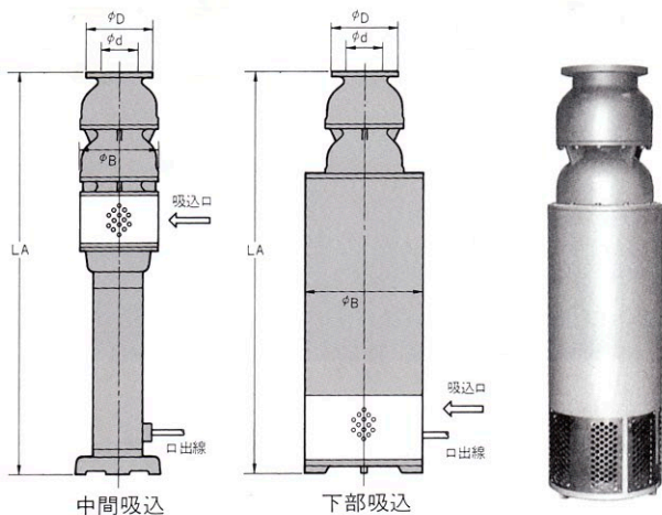
50Hz SSP・USW 選定図 4極
